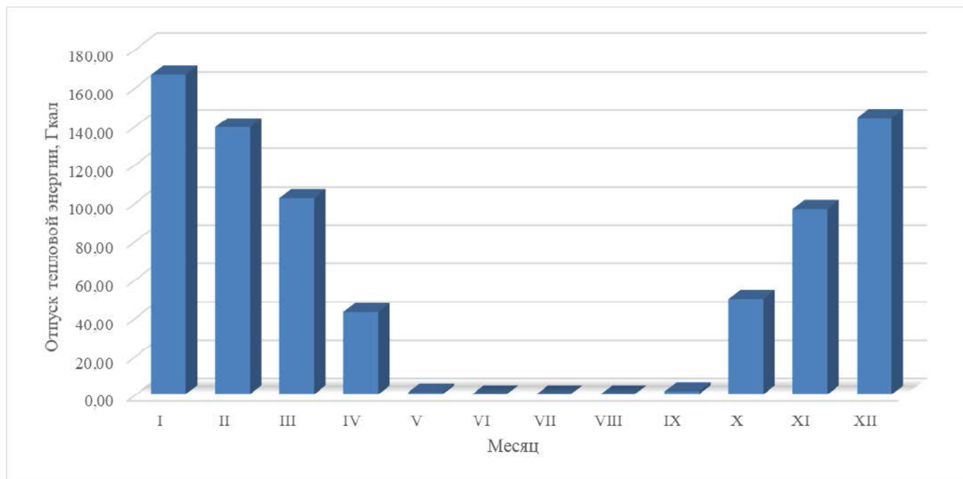
Рисунок 1.3 – Оптимальный температурный график отпуски тепловой энергии по котельной с. Протопоповка
